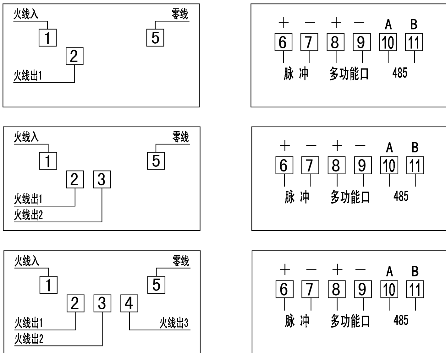
图 7 电能表接线端子功能示图
